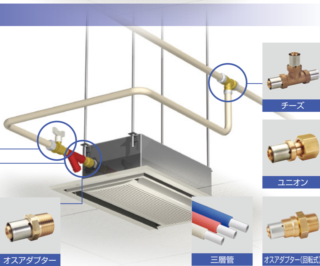
三層管
